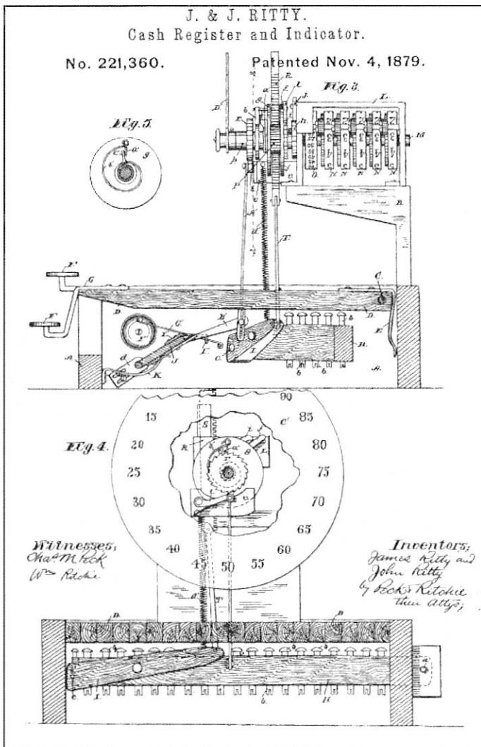
Kasregisteroctrooiaanvraag – J. & J. Ritty - Cash register and indicator – No. 221,360 – Patenred Nov. 4, 1879
